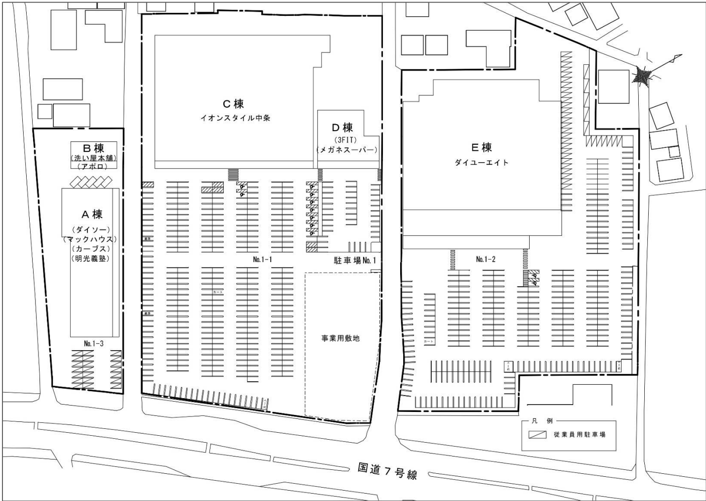
配置図（変更後）
